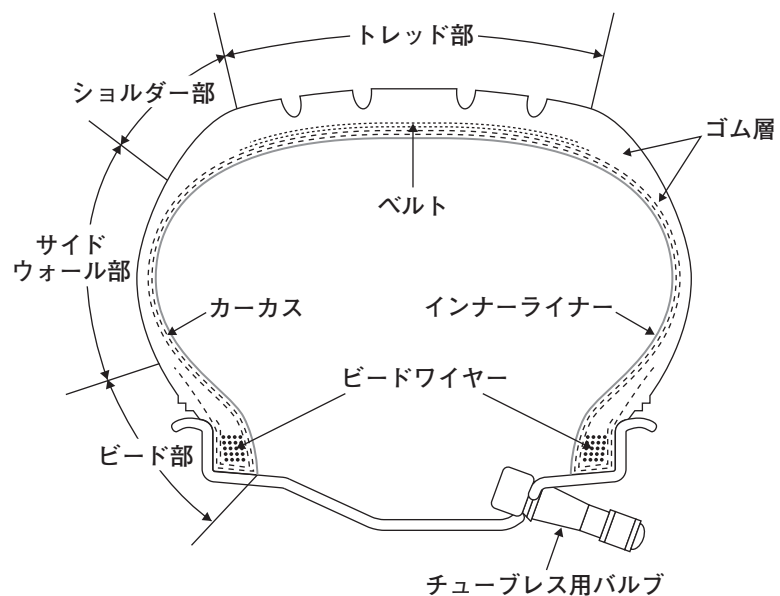
構造部分の名称
