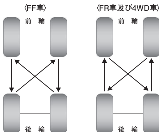
【図7】乗用車用タイヤの位置交換例
