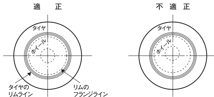
【図13】 ビードシーティングの状態（側面図）
