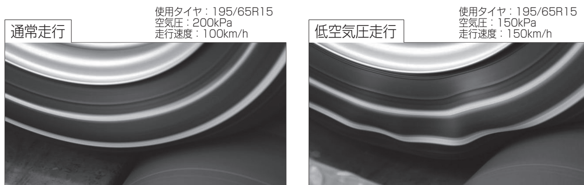
【図5】 スタンディングウェーブ 空気圧不足の状態では高速走行した場合に生じるスタンディングウェーブ現象
