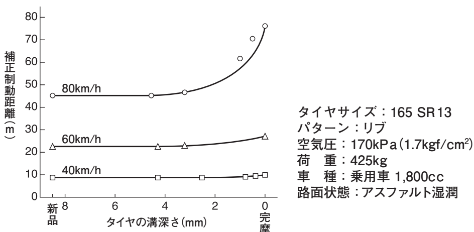
【図10】 ハイドロプレーニング
