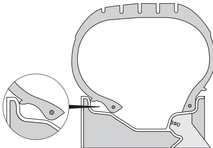
【図12】 不適正なビードシーティング（断面図）
