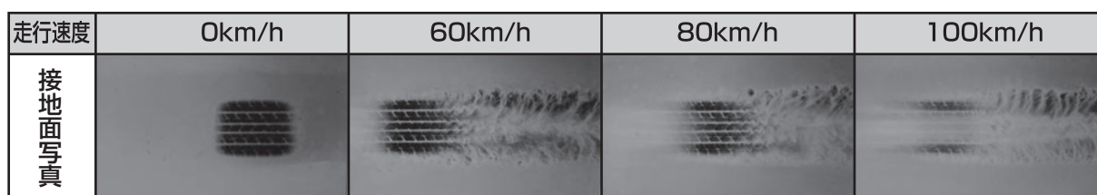
【図10】 ハイドロプレーニング
