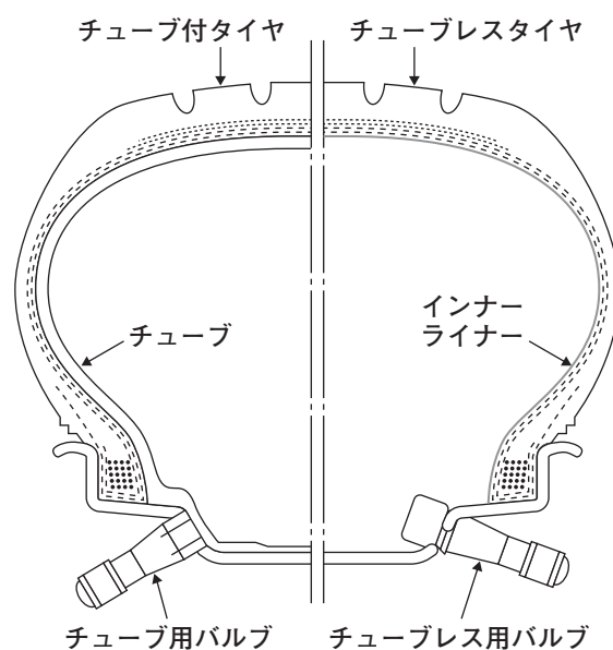
チューブ付タイヤとチューブレスタイヤ
