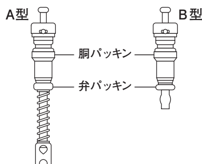
【図2】バルブコアの種類
