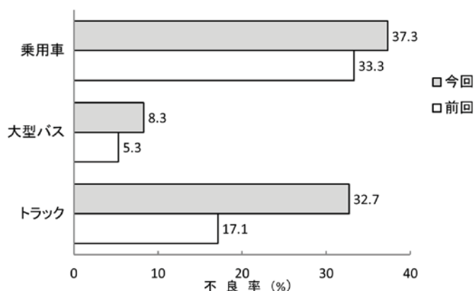
図-1 車種別・タイヤ整備不良率の比較
